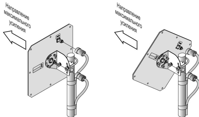
Рисунок 2. Сборка антенны
