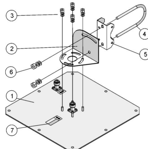
Рисунок 2. Сборка антенны
