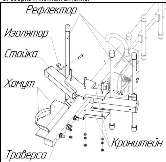
Схема 1 – Сборка антенны
