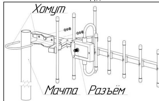
Схема 2 – Монтаж антенны на мачте
