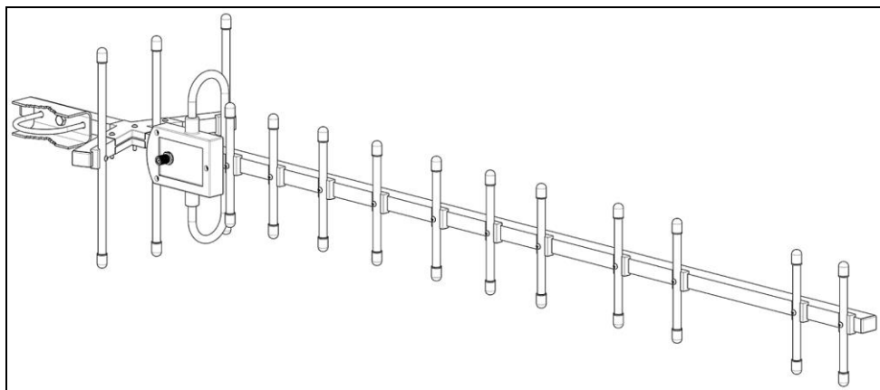
Рисунок 2 – Внешний вид собранной антенны
